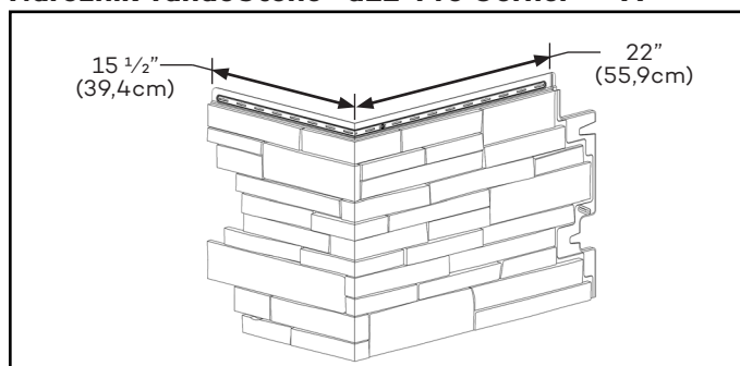
Narożnik TandoStone® aLL-Pro Corner® - "A"
